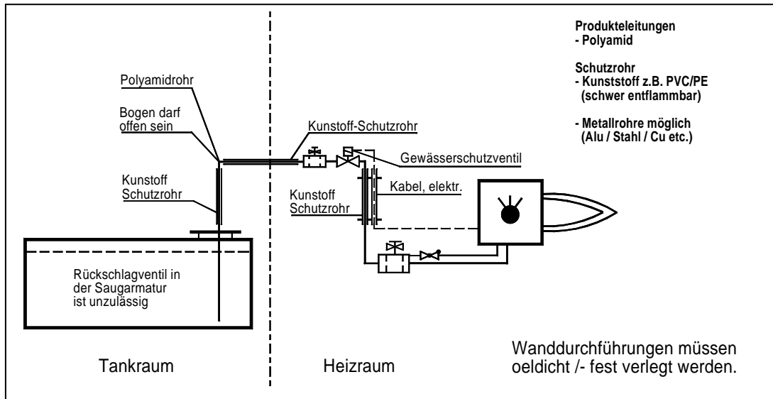
Verlegungsart: Installation ohne Fremdraum
