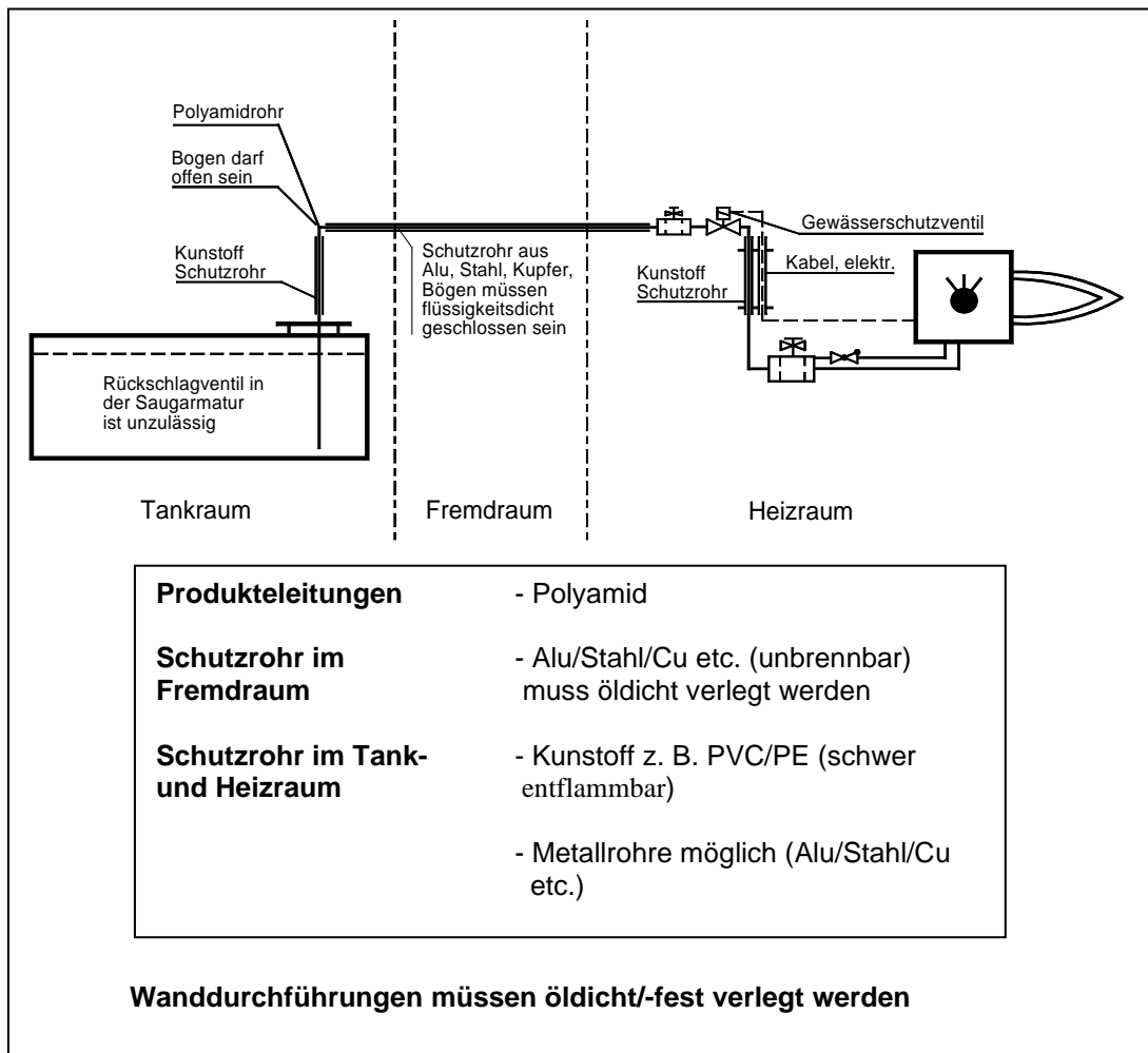
Verlegungsart: Installation durch Fremdraum
