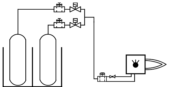
Anlage gilt als ein Behälter
