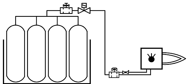
Anlage gilt als ein Behälter
